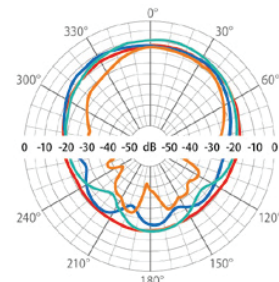
Suuntaavuuskaavio
